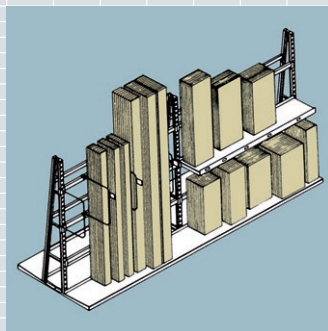
Vertikální regály OHRA – materiály jsou po ruce
