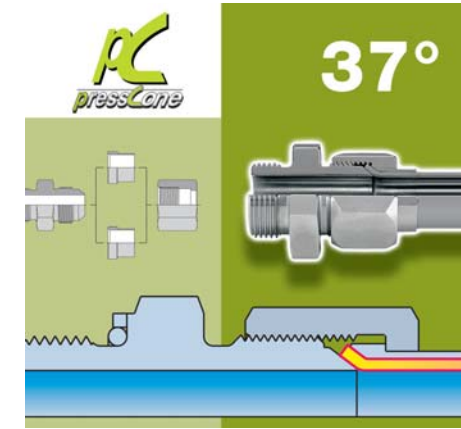
šroubení JIC – 37° 37° JIC Fittings
